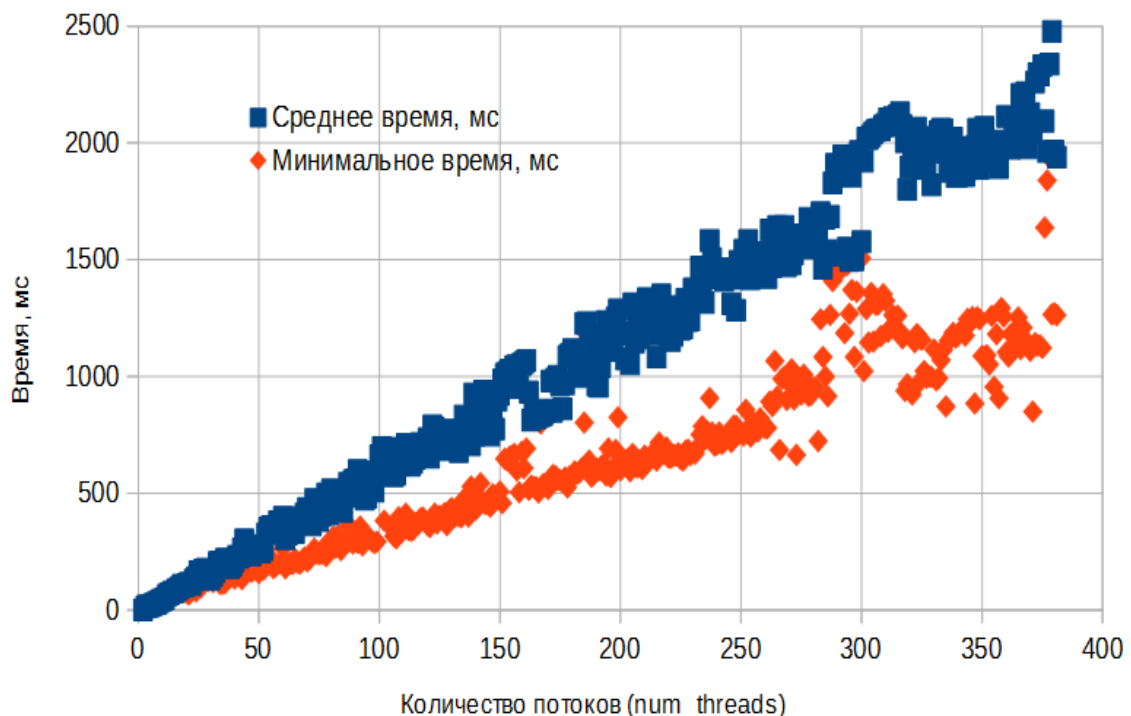
Рисунок 3 – Результаты измерения накладных расходов OpenMP при создании и удалении потоков
