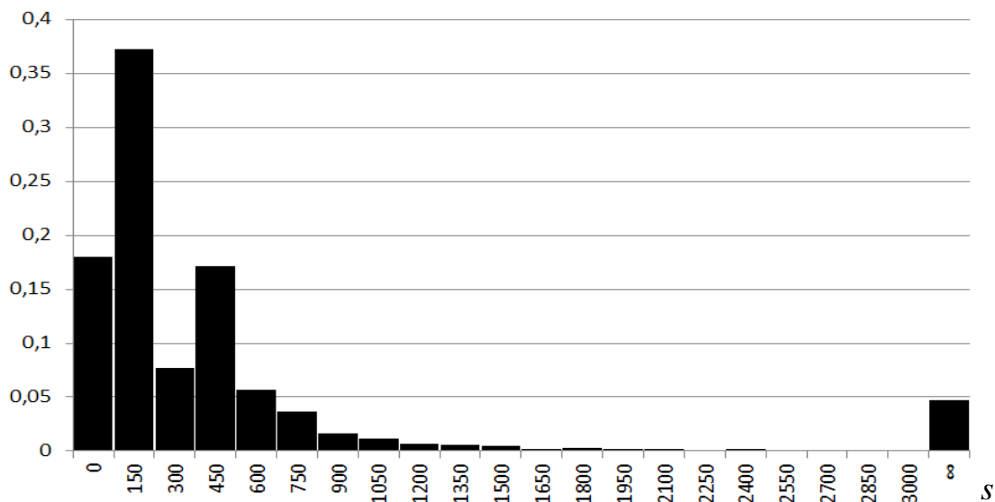
Рисунок 4 – Гистограмма распределения количества запусков параллельной программ до возникновения взаимоблокировки
