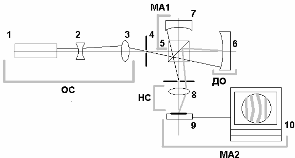
Рис. 4. Принципиальная схема установки контроля сферического зеркала на неравноплечем лазерном интерферометре
