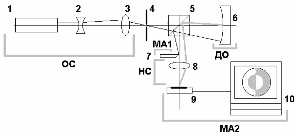
Рис. 2. Принципиальная схема установки контроля сферического зеркала теньвым методом
