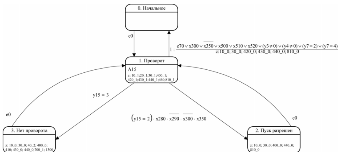
Рисунок 2. Граф переходов
