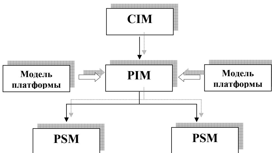
Рисунок 4. Схема взаимодействия
