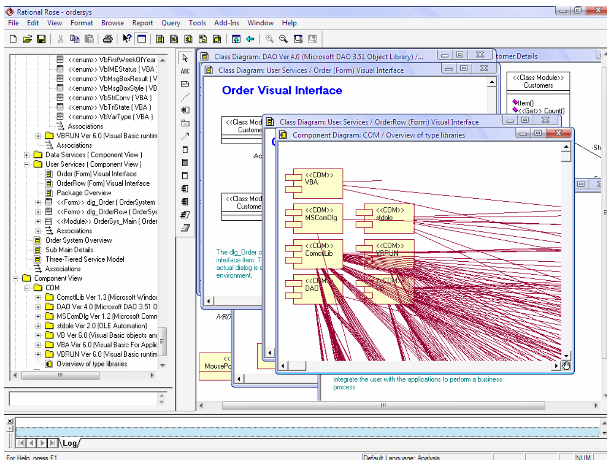
Рисунок 10. Диаграмма компонентов
