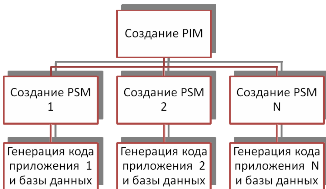
Рисунок 3. Создание MDA-приложений
