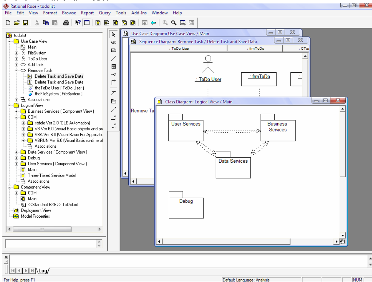
Рисунок 6. Диаграмма классов
