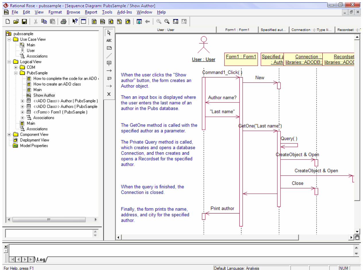
Рисунок 9. Диаграмма сценариев
