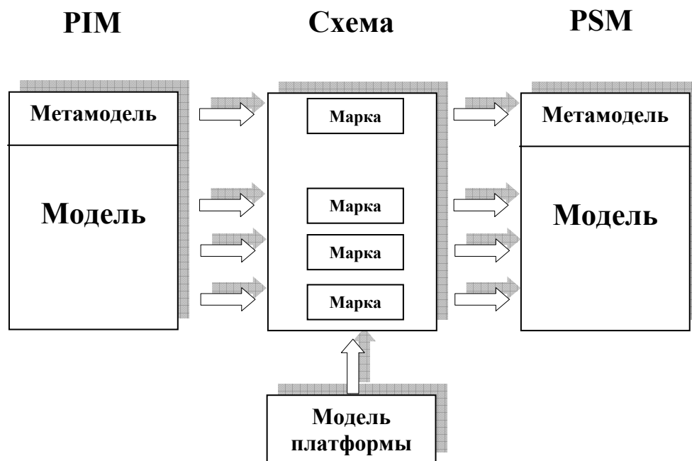
Рисунок 5. Модель платформы
