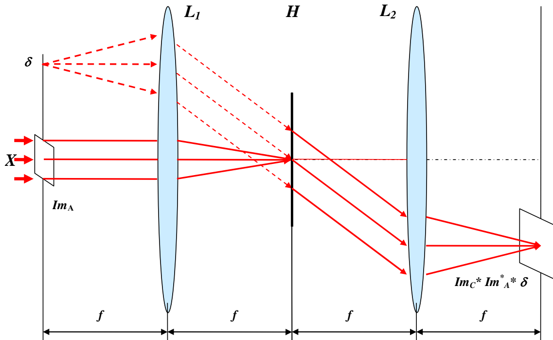
Рис.3.2. Схема голографического коррелятора Ван дер Люгта
