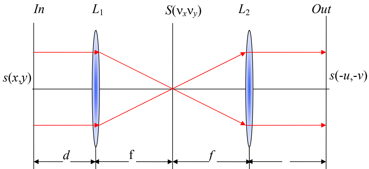
Рис.1.4. Схема двойного оптического преобразования Фурье
