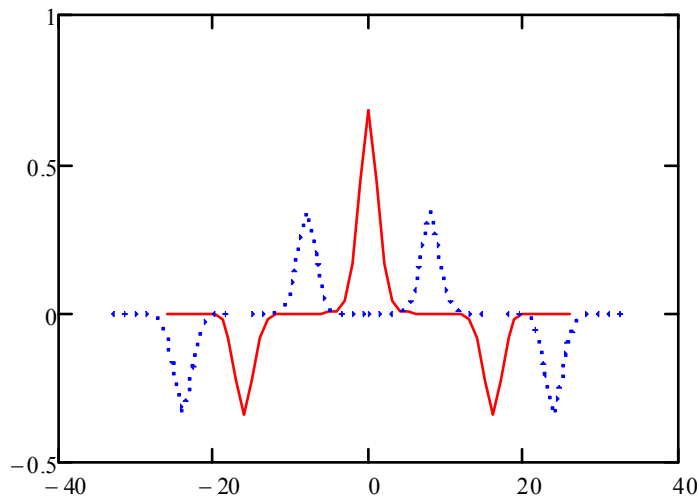
Рис.2.4. Функции автокорреляции (сплошная кривая) и кросс-корреляции дифференцированных изображений
