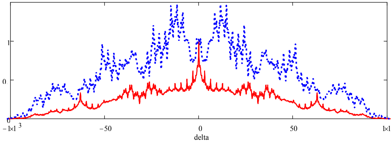
Рис.3.3. АКФ (сплошная линия) и ВКФ (пунктир)
