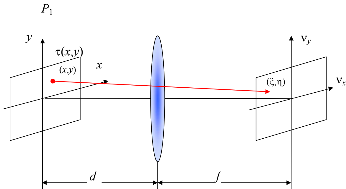
Рис.1.1. Схема, реализующая двумерное преобразование Фурье
