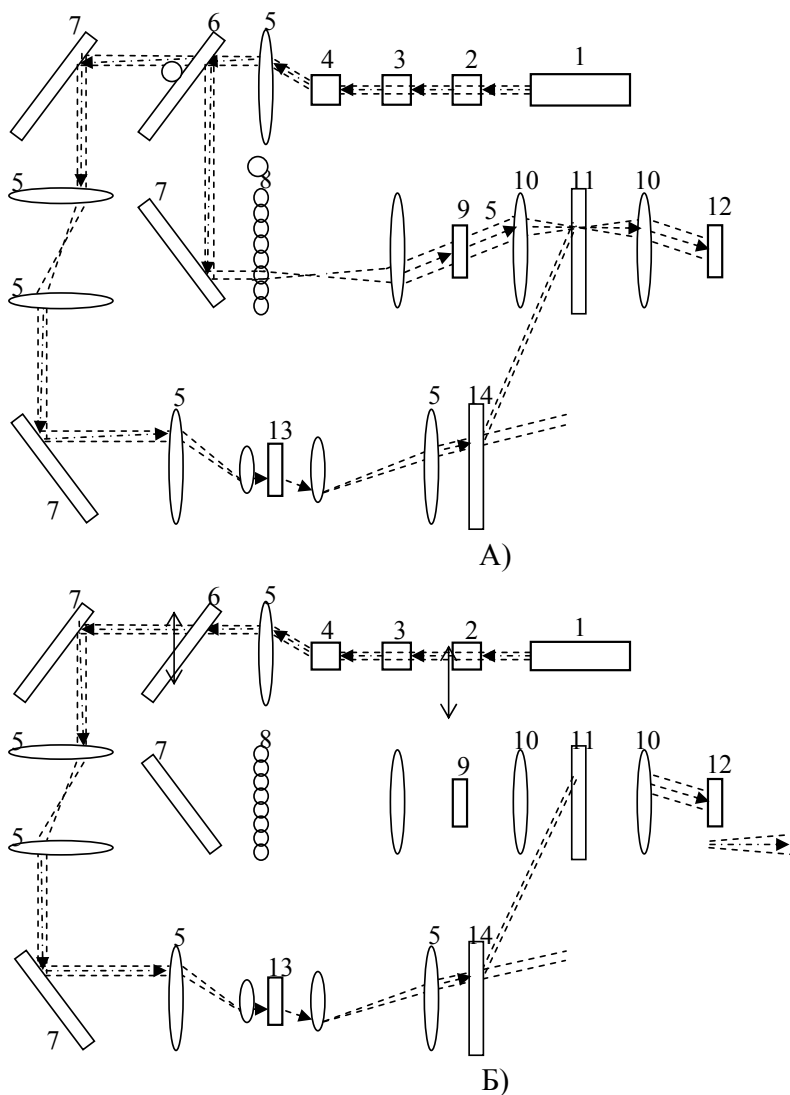
Рис.17. Оптическая схема реализации голографической памяти с изменяющимся углом падения опорного пучка в объемной среде в режиме записи (А) и считывания (Б) информации.
