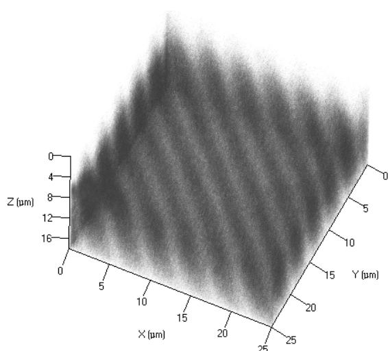
Рис.37. Микрофотография фрагмента объёмной голограммы * с пространственной частотой 300 \text{ мм}^{-1} , записанной в полимерном материале с фенантренхиноном. Интенсивность окраски тёмных участков соответствует концентрации продуктов фотоприсоединения ФХ к полимеру; изображение получено с помощью конфокального сканирующего микроскопа Zeiss LSM 710.
