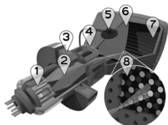
Рис.41. Устройство современного ЭЛТ дисплея:
