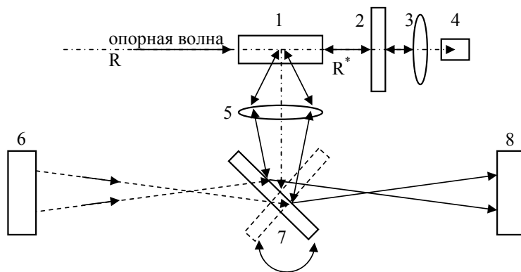
Рис.18. Оптическая схема, реализующая восстановление голограммы комплексно-сопряженным опорным пучком.
