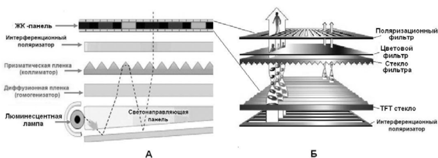
Рис.42. Структура (А) и принцип действия (Б) ЖК дисплея
