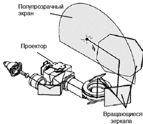
Рис.47. Структурная схема объемного 3D-дисплея Perspecta 1.9.
