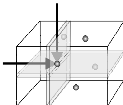
Рис.3. Принцип двухфотонной адресации в объёмной среде: один из световых пучков выделяет слой материала, другой – точку в этом слое; происходит обращение (запись или чтение) к точке, на которую пучки действуют одновременно, то есть в которой они пересекаются. Такой механизм адресации предусмотрен, например, для работы с многослойными флуоресцентными дисками. Возможно также не оптическое, а электрическое выделение слоёв с применением электрохромных (меняющих свои оптические свойства – пропускание, отражение – при приложении напряжения) материалов, таких как оксид вольфрама.
