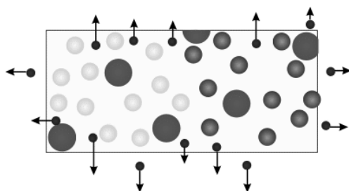
Рис.29. Формирование голограммы в "классическом" реоксоне
