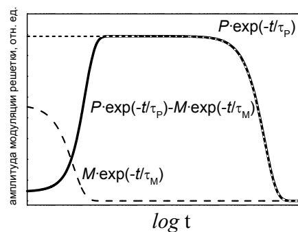
Рис.32. Изменение во времени амплитуд модуляции противофазных периодических распределений (решеток), образованных молекулами исходного рабочего вещества М и его фотопродукта Р с временами жизни \tau_M и \tau_P соответственно, а также амплитуды результирующей решетки (сплошная линия)
