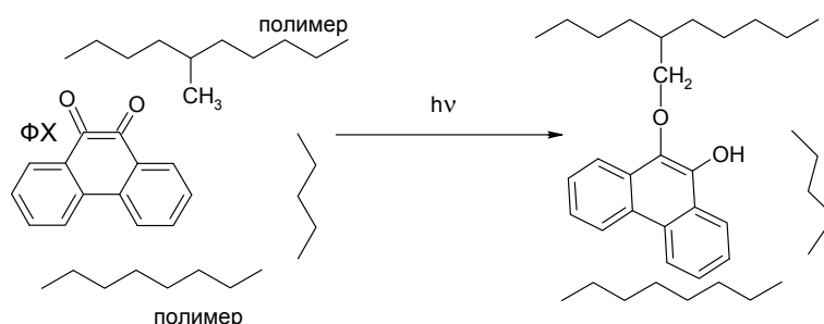
Рис.34. Фотоприсоединение ФХ к макромолекуле
