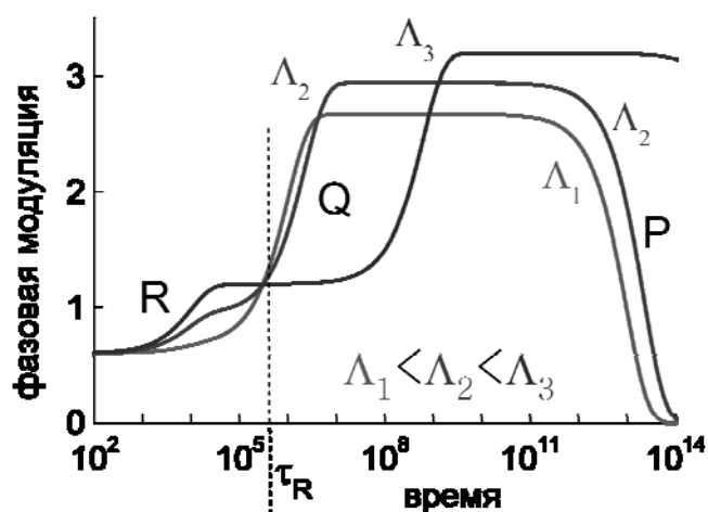
Рис.36. Изменение со временем фазовой модуляции голограмм с пространственными периодами L_1 < L_2 < L_3 , записанных в материале с диффузионным проявлением. Буквами R, Q, P отмечены этапы развития голограмм, на которых основную роль в изменении фазовой модуляции играют соответственно радикалы, ФХ и конечный (стабильный) продукт его трансформаций.
