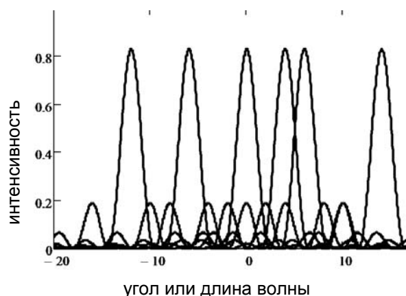
Рис.5. Мультиплексирование голограмм: угловая и связанная с ней спектральная селективность, присущие объёмной голограмме, позволяют реализовать раздельное обращение к различным блокам информации, записанным в одном объёме среды в виде наложенных голограмм, считывая её под разными углами или светом с разными длинами волн (угловое или спектральное мультиплексирование).
