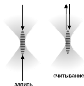
Рис.15. Схема записи и считывания отражательных микроголограмм
