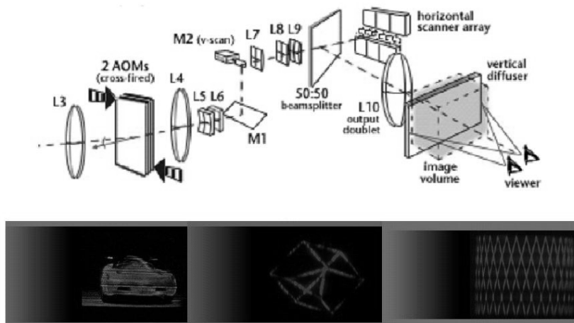
Рис.46. Лабораторный макет голографического 3D-дисплея, созданного в MIT под руководством С. Бентона
