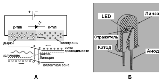
Рис.44. Принцип действия (А) и конструктивное исполнение (Б) светового диода.
