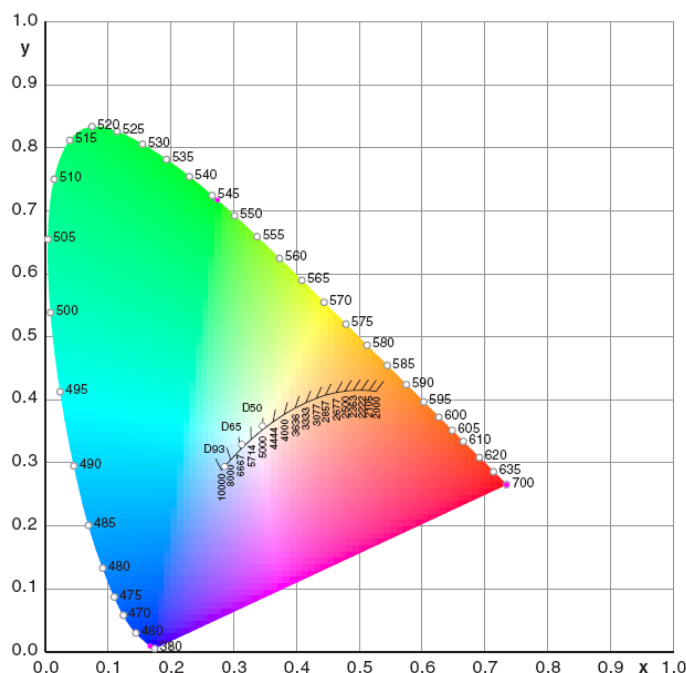
Рис.39. Цветовой «треугольник» МКО 1931 года
