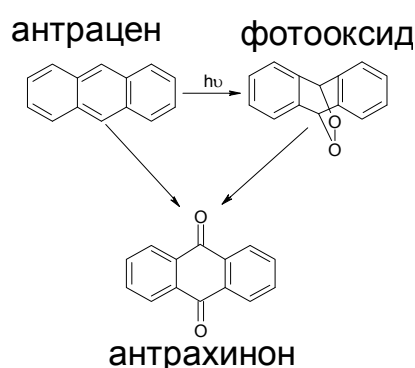
Рис.31. Схема превращений, происходящих в реоксане при записи (фотореакция антрацен-фотооксид) и после неё (темновые трансформации и фотооксида, и антрацена в другие соединения, из которых на схеме условно показан только антрахинон)
