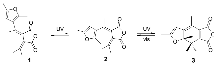
Рис.22. Схема фотохромных превращений фульгидного красителя, включающая переходы между бесцветными (не поглощающими в видимой области) открытыми формами 1 и 2 и между формой 2 и окрашенной замкнутой формой 3 .
