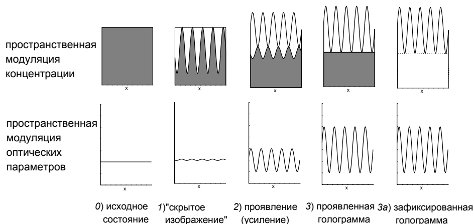
Рис.35. Пояснение к механизму формирования голограммы в материале с фенантрехиноном
