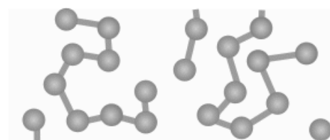
Рис.25. Схема формирования голограмм в фотополимерах без нейтральных компонент
