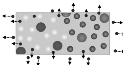
Рис.30. Формирование голограмм в реоксане со световым проявлением.
