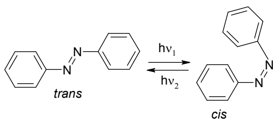
Рис.21. Типичный фотохромный процесс – обратимая транс-цис фотоизомеризация азобензола
