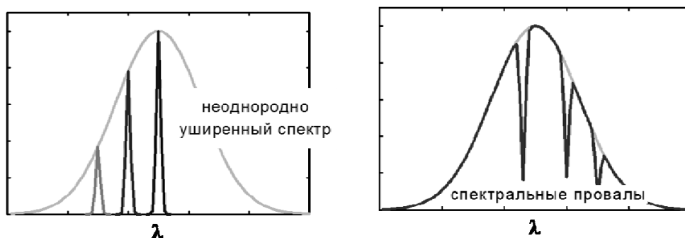
Рис.4. Реализация собственной спектральной селективности материала для оптической памяти за счёт выжигания стабильных спектральных провалов (persistent spectral hole burning). При воздействии узкополосного лазерного излучения на спектр ансамбля молекул, неоднородно уширенный до 1 ГГц – 10 ТГц из-за взаимодействия со средой при неэквивалентности различных пространственных локализаций, селективно возбуждаются подансамбли молекул, поглощающих узкополосное возбуждающее излучение, таким образом из широкого спектра изымаются узкие (100 Гц) полосы.
