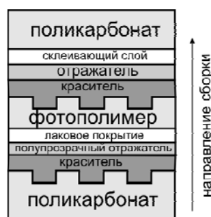
Рис.9. Структура двуслойного диска DVD-R (без соблюдения масштаба толщины). На рисунке показана половина диска. Двусторонний двуслойный диск состоит из двух таких половин, в одностороннем половине толщины занята поликарбонатной подложкой. Запись и считывание информации производятся снизу.
