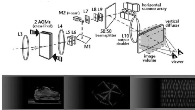
Рис.46. Лабораторный макет голографического 3D-дисплея, созданного в МИТ под руководством С. Бентона
