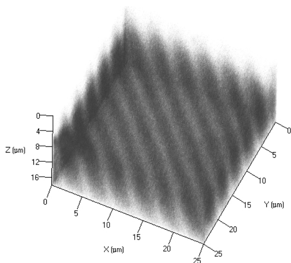
Рис.37. Микрофотография фрагмента объёмной голограммы* с пространственной частотой 300 \text{ мм}^{-1} , записанной в полимерном материале с фенантренхиноном. Интенсивность окраски тёмных участков соответствует концентрации продуктов фотоприсоединения ФХ к полимеру; изображение получено с помощью конфокального сканирующего микроскопа Zeiss LSM 710.
