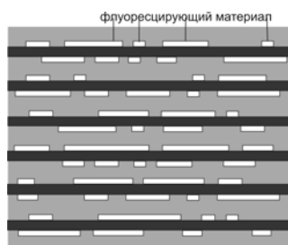
Рис.14. Структура многослойного флуоресцентного диска
