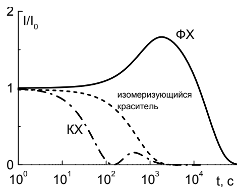
Рис.33. Возможные формы кривых постэкспозиционной релаксации фотоиндуцированных решёток (проявление эффекта дополнительных решёток на примерах ФХ, камфорхинона и изомеризирующегося красителя в низкомолекулярном стекле):
