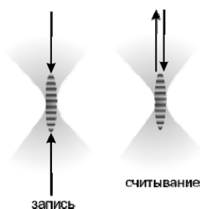
Рис.15. Схема записи и считывания отражательных микроголограмм
