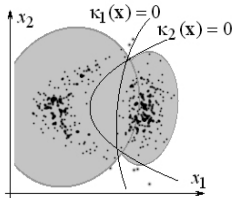
Рис. 31. Пример решения задачи распознавания для двух классов, разделимых кривой второго порядка k_2(\mathbf{x}) = 0 ; использование метода максимального правдоподобия и описание распределения образов каждого из классов с помощью нормального закона приводит к построению разделяющей границы, которая также описывается кривой второго порядка k_1(\mathbf{x}) = 0 , но не является оптимальной
