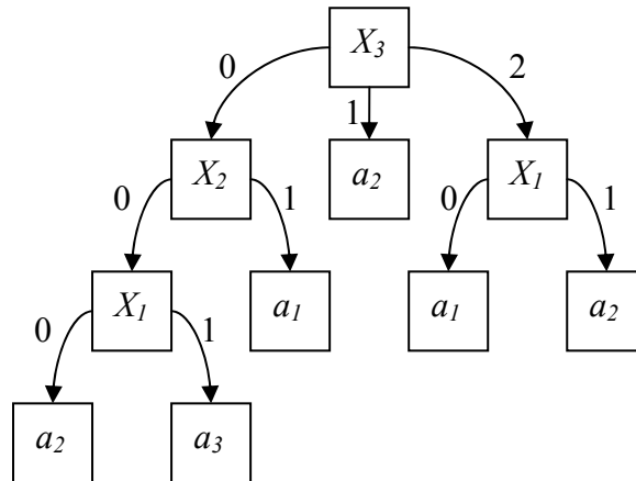
Рис. 50. Дерево решений, строящееся алгоритмом ID3 при выборе наиболее информативных признаков
