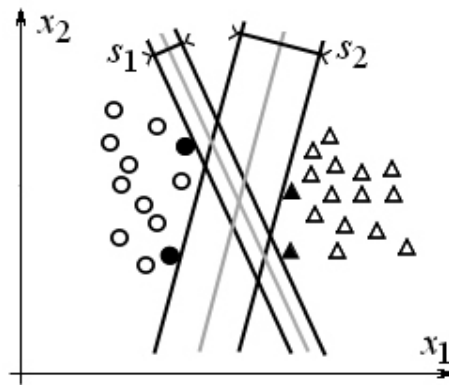
Рис. 28. Два линейно разделяемых класса образов, для которых представлены две разделяющие полосы с разными ширинами: s_1 и s_2
