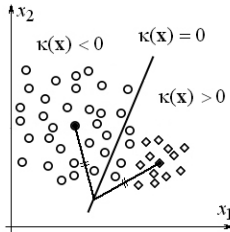
Рис. 26. Пример двух классов разных размеров, для которых критерий евклидова расстояния до эталонных образов не является корректным
