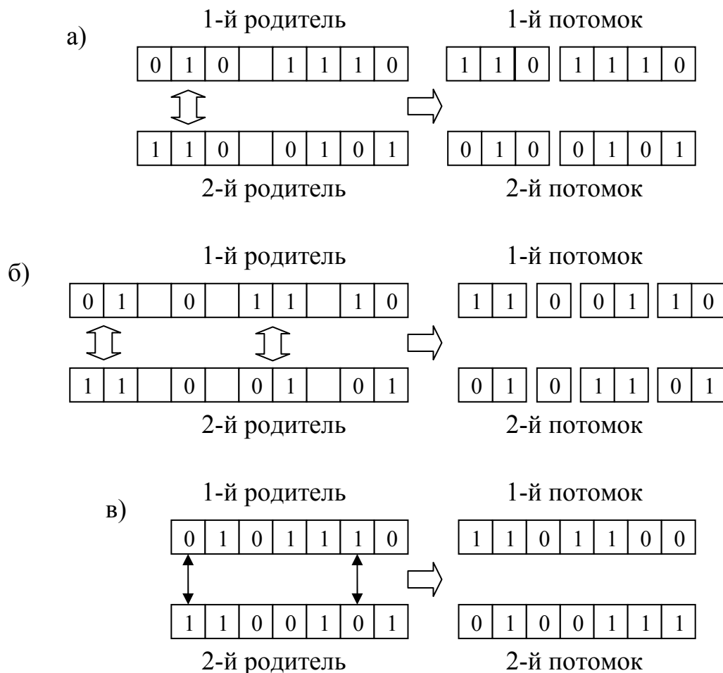
Рис. 8. Примеры работы оператора скрещивания: а) одноточечного; б) многоточечного; в) обмена случайными битами
