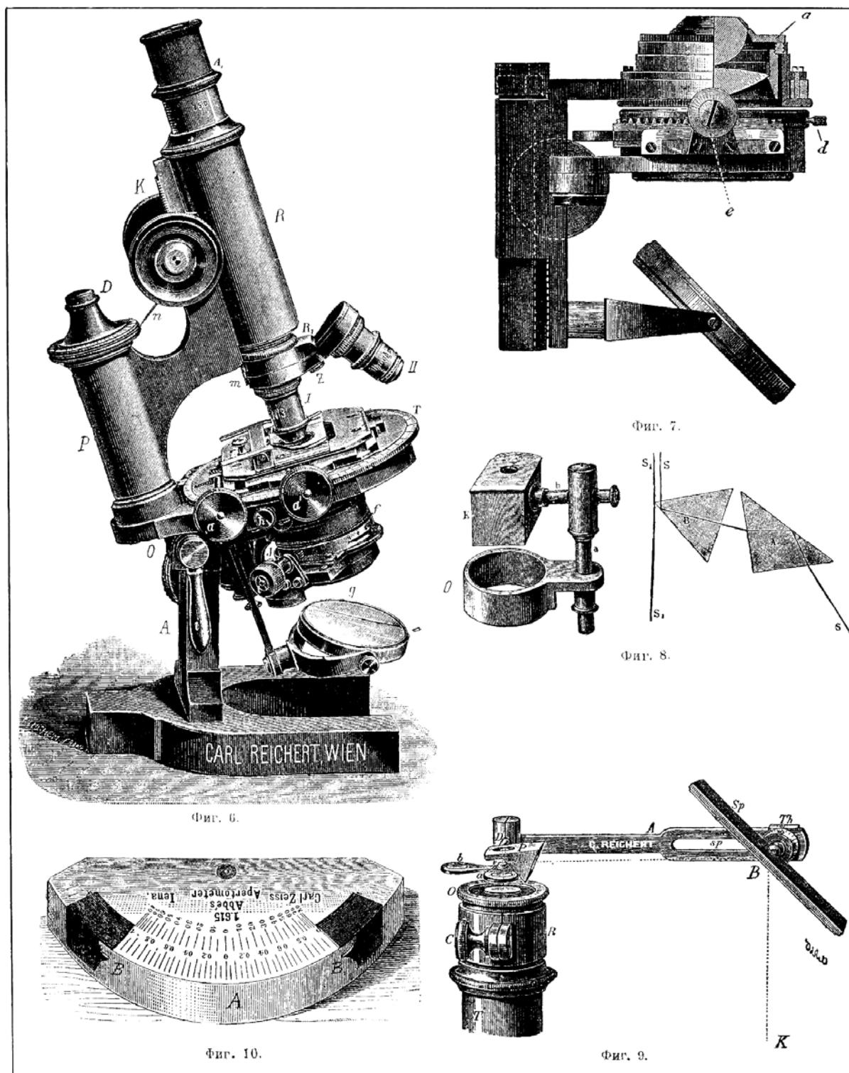
Фиг. 6. Микроскопъ съ объективнымъ револьверомъ и конденсаторомъ Аббе. Фиг. 7. Конденсаторъ Аббе. Фиг. 8 и 9 Приборы для рисования и опредѣленія увеличенія. Фиг. 10. Апертометръ Аббе.
