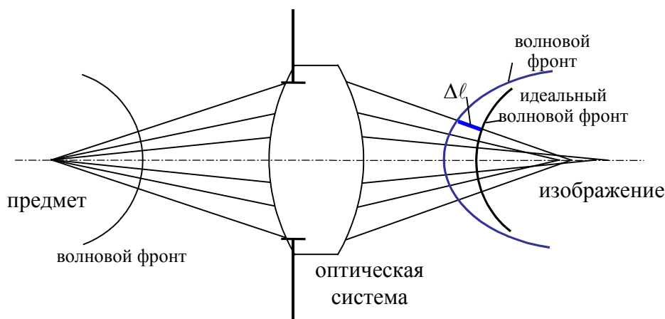
Рис. 3.7. Волновая aberrация
