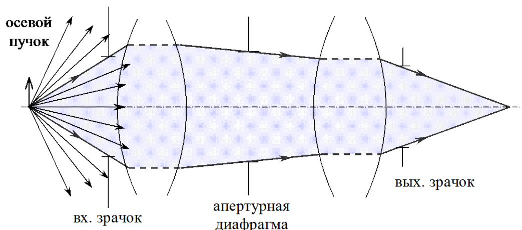
Рис. 3.2. Апертурная диафрагма
