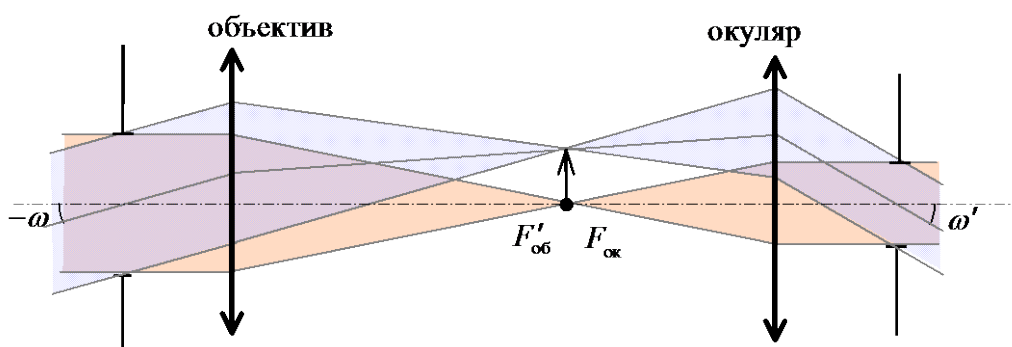
Рис. 5.1. Телескопическая система
