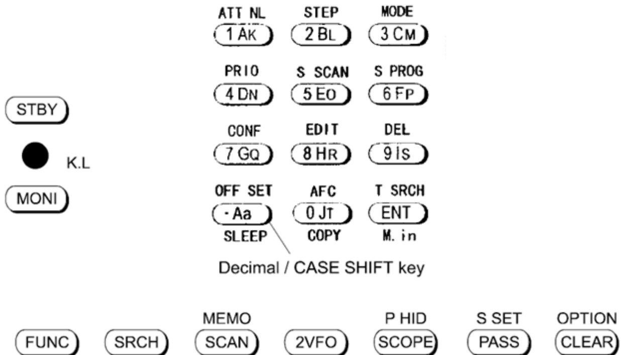
Рис.19. Клавиатура AR8600
