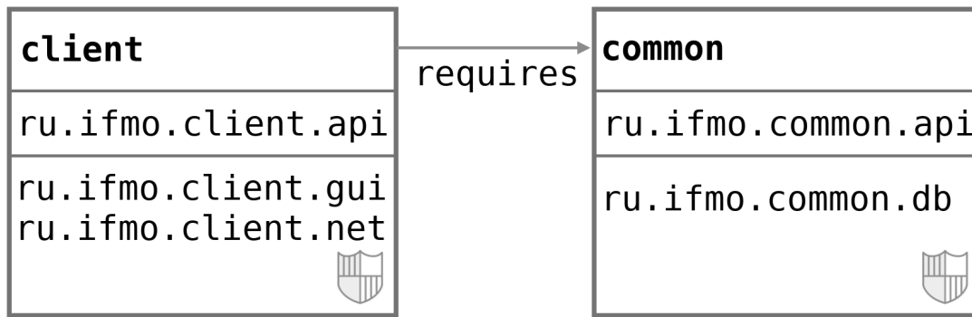
Рисунок 2. Взаимосвязанные модули
