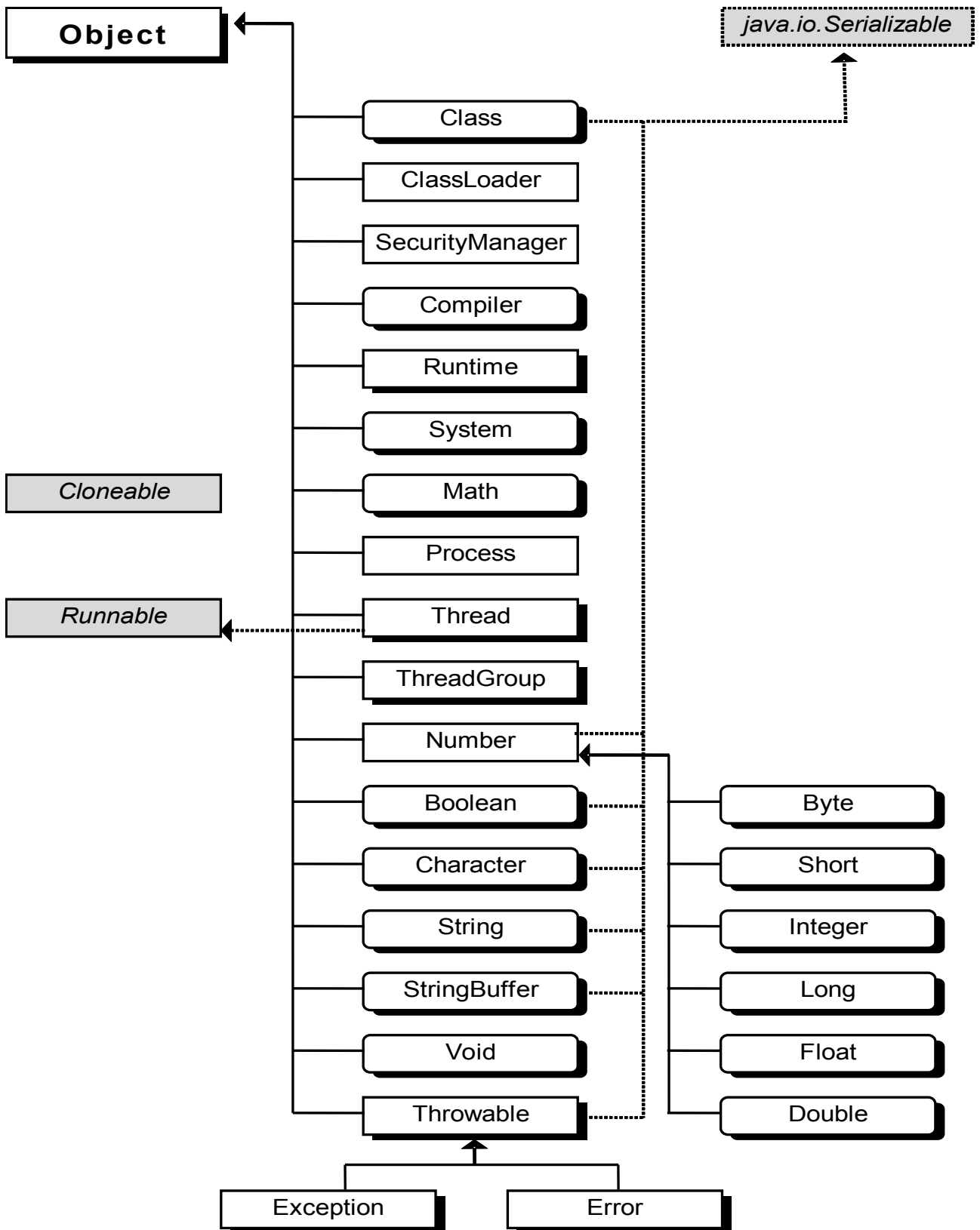
Рисунок 3. Пакет java.lang
