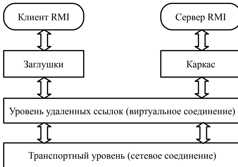
Рисунок 9. Структура RMI
