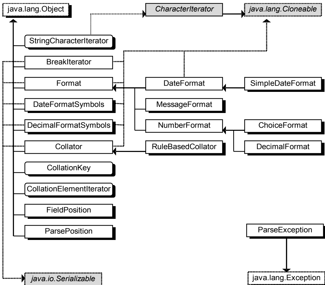
Рисунок 10. Пакет java.text.
