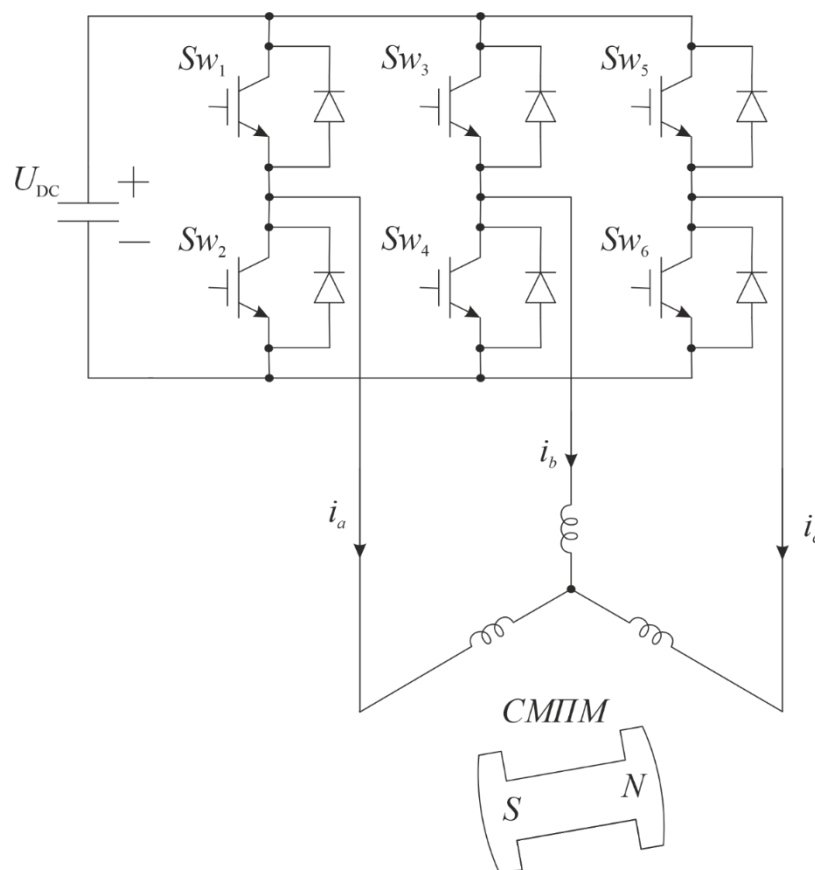
Рисунок 1.1 – Трехфазный ШИМ инвертор с синхронной машиной с постоянными магнитами.
