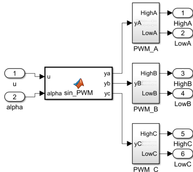
Рисунок 1.4 – Блок «Switch Control System», реализующий синусоидальную ШИМ.
