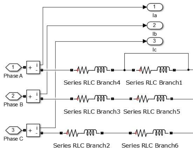
Рисунок 2.6 – Блок «Inverter with PMSM» при межвитковом замыкании в фазе А.
