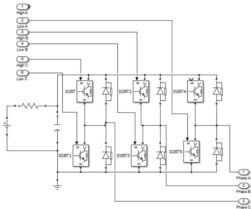
Рисунок 2.2 – Блок «Inverter with PMSM» при выходе из строя канала управления верхним ключом в фазе А.
