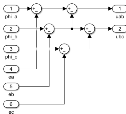
Рисунок 1.11 – Блок «Linear Voltages».
