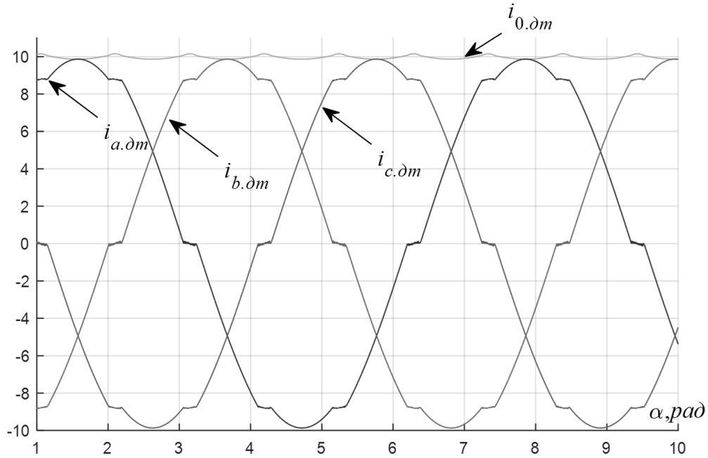
Рисунок 3.3 – Графики токов СМППМ и обобщенного тока i_{0.cs} при идентификации параметров K_{об.дм} и \tau по результатам эксперимента с изменением параметра \alpha .
