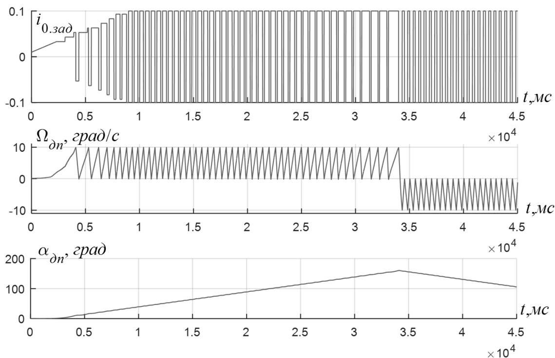
Рисунок 6.4 – Графики задания на контур тока i_{0.zad} , скорости вращения электропривода \Omega_{\partial n} и угла поворота ротора \alpha_{\partial n} при получении экспериментальных данных для идентификации параметров электропривода.
