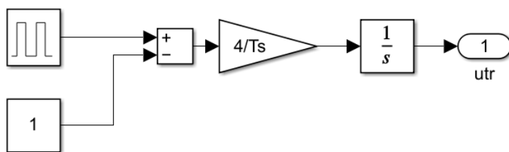
Рисунок 1.2 – Блок генератора пилообразного сигнала «Triangle Wave».
