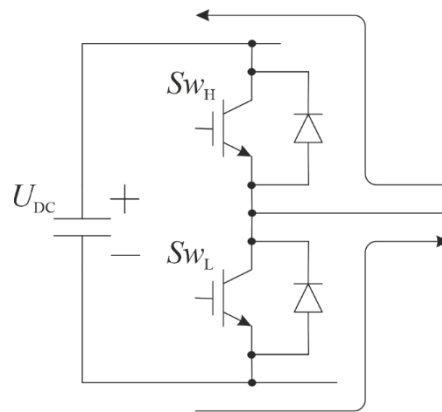
Рисунок 1.14 – Направление протекания тока в течение «мертвого времени» в одной из стоек трехфазного инвертора.
