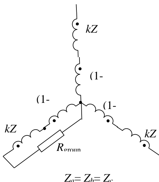
Рисунок 2.9 – Замыкание фазы А статорной обмотки двигателя на корпус.
