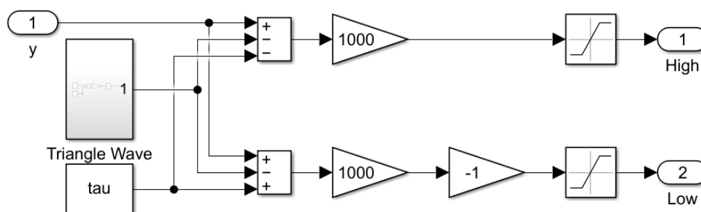
Рисунок 1.8 – Блок «PWM» с «мертвым временем».
