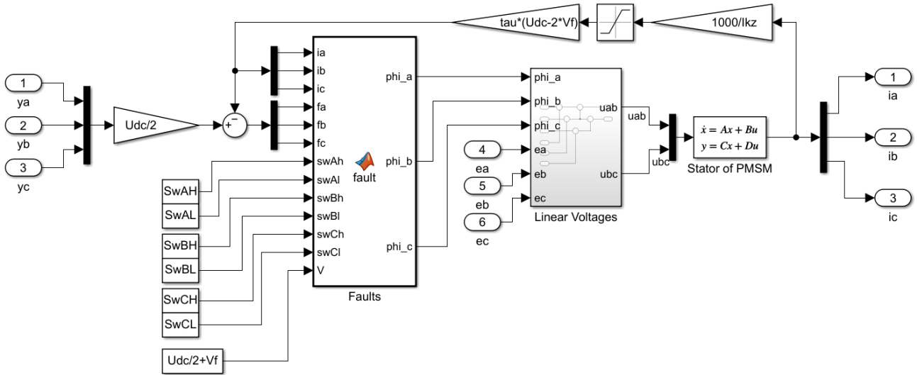
Рисунок 2.12 – Блок «Inverter with PMSM», реализующий аналитическую модель инвертора с СМПИМ в виде дифференциальных уравнений, при выходе из строя верхнего транзистора в стойке инвертора в фазе А.
