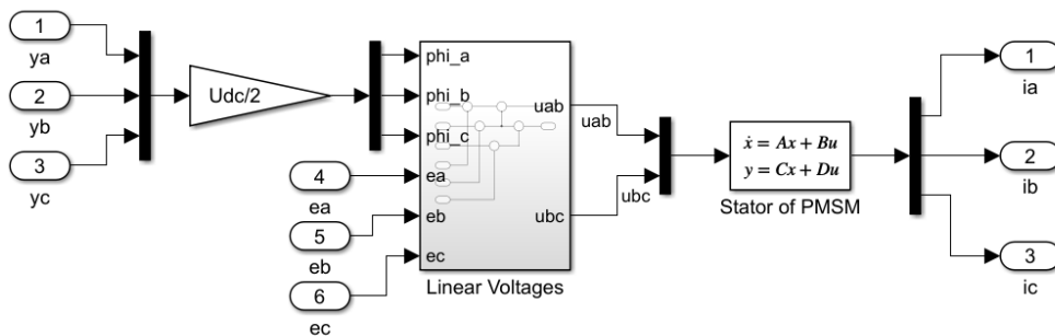
Рисунок 1.10 – Блок «Inverter with PMSM».
