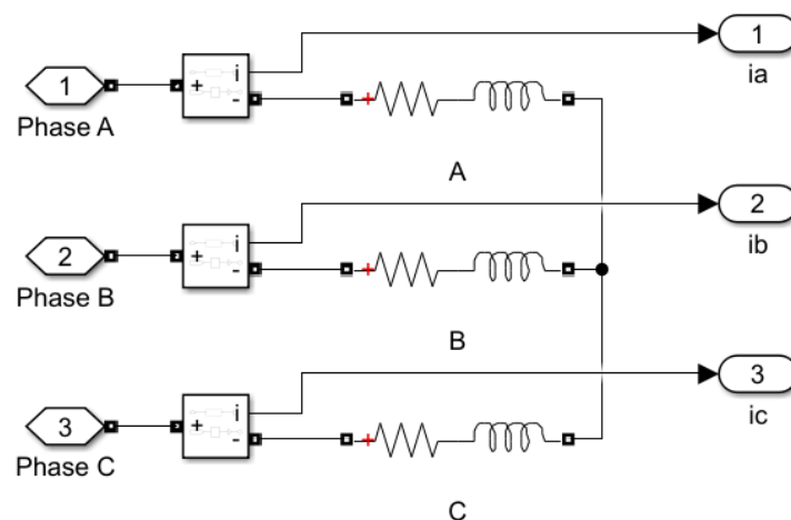
Рисунок 1.6 – Блок «Stator of PMSM», реализующий модель статорной обмотки СМПМ без учета противо-ЭДС.
