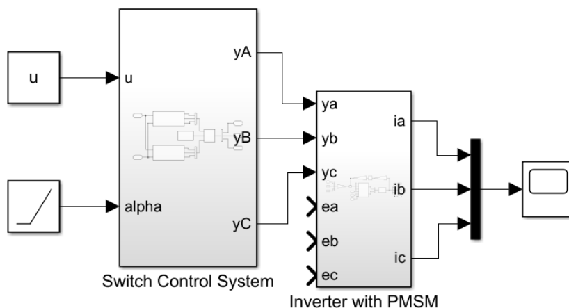
Рисунок 1.13 – Блок трехфазного ШИМ инвертора с подключенной СМПМ.
