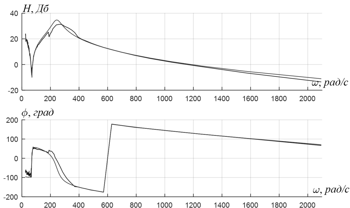
Рисунок 6.11 – Экспериментальные ЛАЧХ H(\omega) и ФЧХ \varphi(\omega) электропривода без сухого трения (светло-серый график) и при наличии сухого трения и релейного регулятора скорости (темно-серый график).
