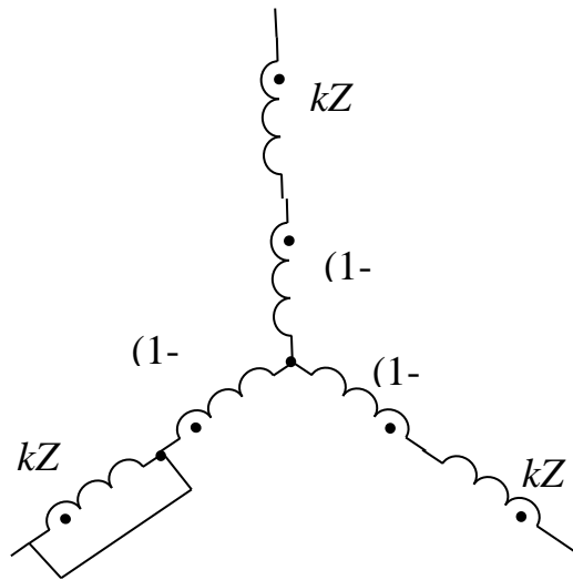
Рисунок 2.5 – Межвитковое замыкание в фазе А.
