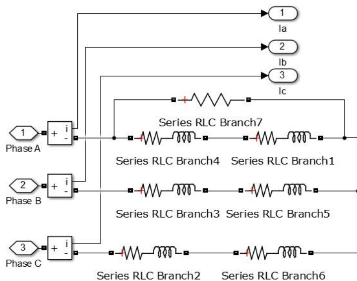
Рисунок 2.10 – Блок «Inverter with PMSM» замыкания фазы А статорной обмотки двигателя на корпус.
