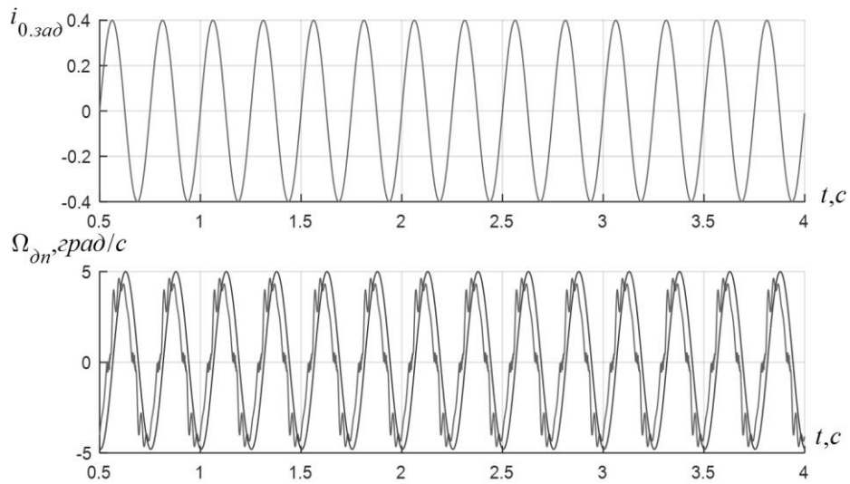
Рисунок 6.7 – Графики задания на контур тока i_{0.zad} и скорости ротора \Omega_{\partial n} во время эксперимента в системе без сухого трения (темно-серый график) и в системе с сухим трением (светло-серый график).
