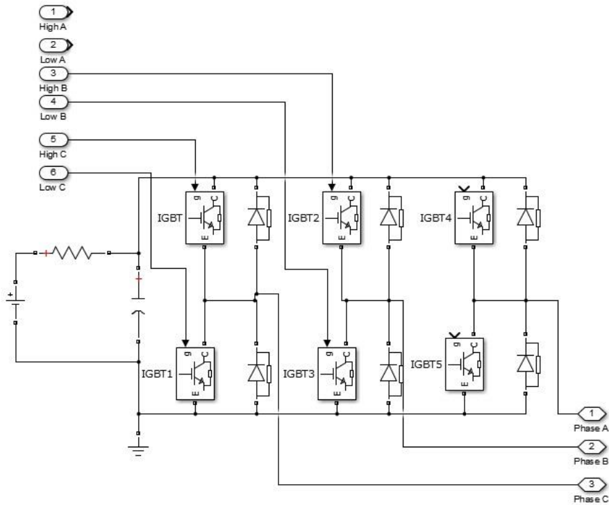
Рисунок 2.4 – Блок «Inverter with PMSM» при выходе из строя каналов управления обоими ключами в фазе А.
