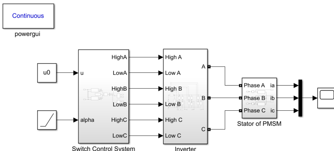
Рисунок 1.7 – Модель трехфазного ШИМ инвертора с подключенной СМПМ реализованная средствами библиотеки SimPowerSystems .
