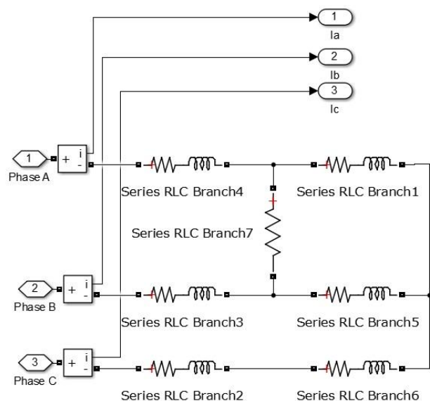
Рисунок 2.8 – Блок «Inverter with PMSM» при межфазном замыкании между фазами А и В.
