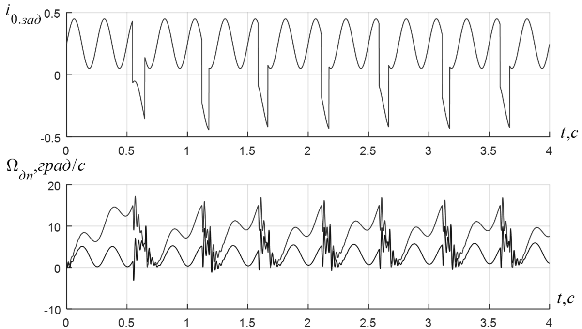
Рисунок 6.10 – Графики задания на контур тока i_{0.zad} и скорости ротора \Omega_{0n} во время эксперимента с релейным регулятором.
