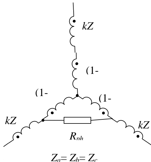
Рисунок 2.7 – Межфазное замыкание между фазами А и В.
