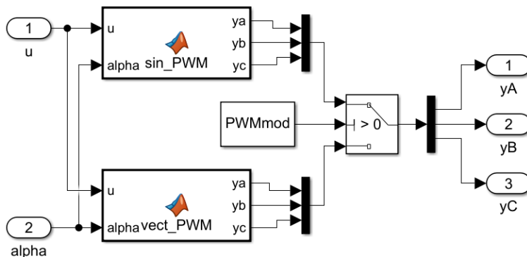
Рисунок 1.12 – Блок «Simple Switch Control System».
