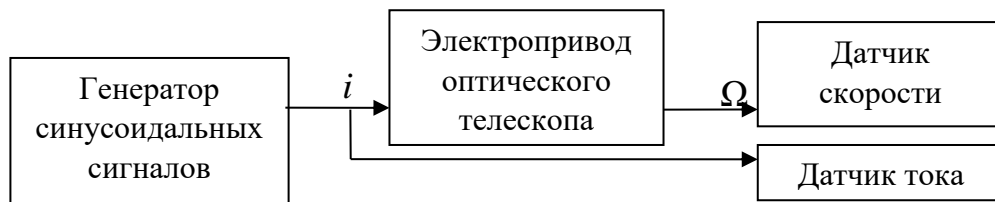
Рисунок 6.6 – Структурная схема эксперимента идентификации частотной характеристики электропривода оптического телескопа.
