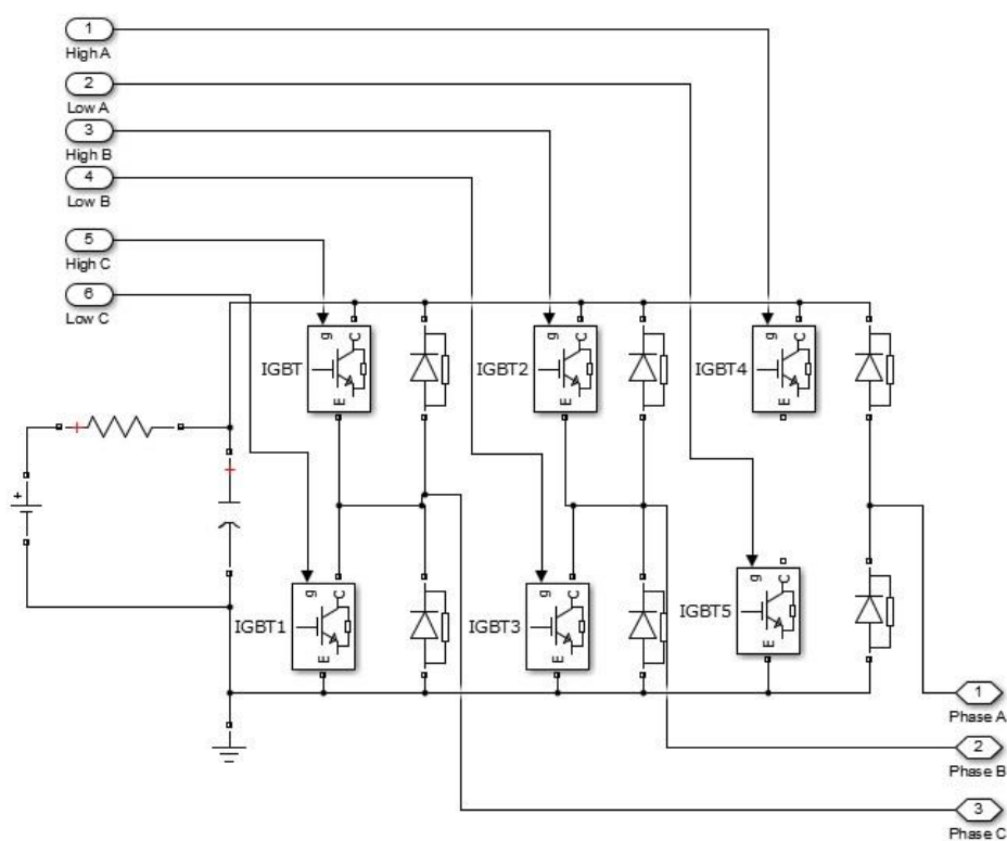
Рисунок 2.3 – Блок «Inverter with PMSM» при выходе из строя обоих транзисторов в фазе А.
