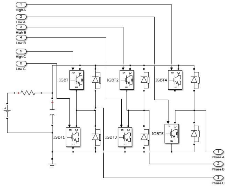
Рисунок 2.1 – Блок «Inverter with PMSM» при выходе из строя верхнего транзистора в фазе А.
