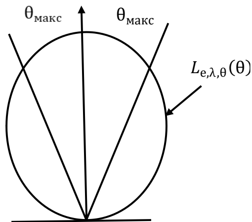
Рисунок 3.7 – Возможная модель пространственного распределения яркости L_{e,\lambda,\theta}(\theta) излучения реальных источников
