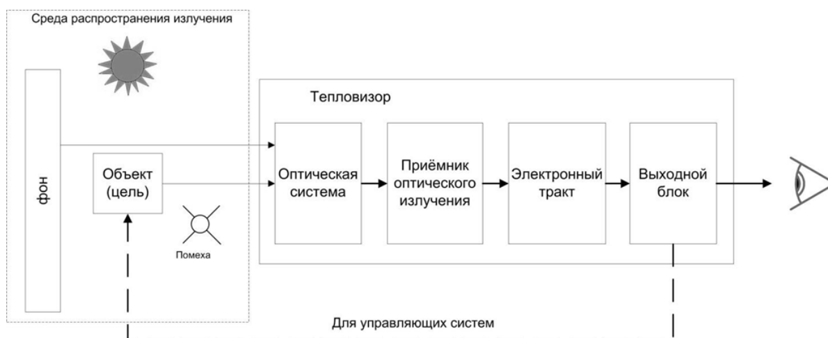
Рисунок 1.1 – Обобщённая структурная схема оптико-электронного прибора
