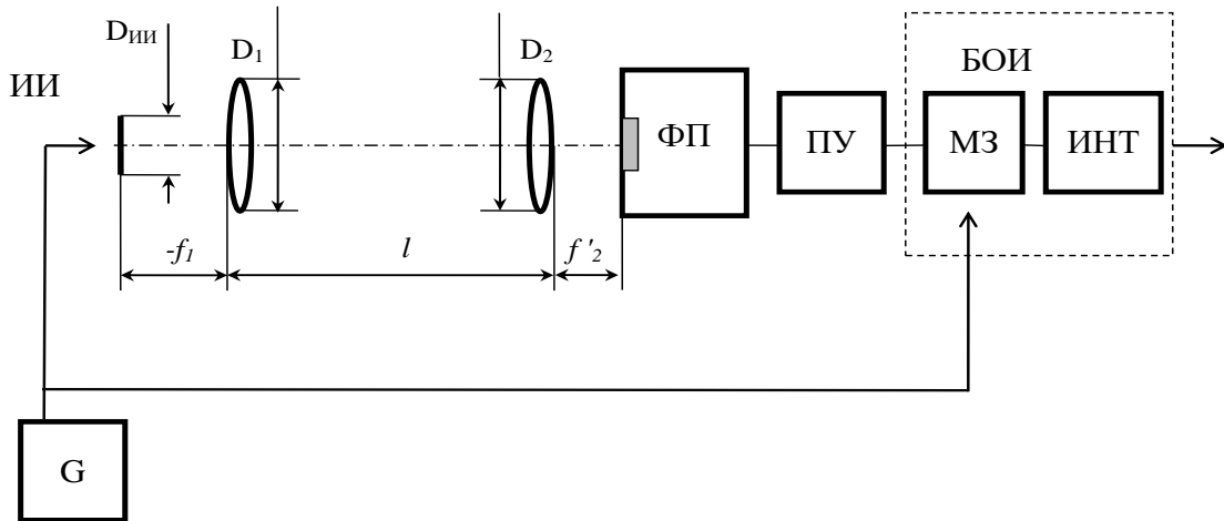
Рисунок 8.1 – Схема коллимационного опико-электронного прибора:
