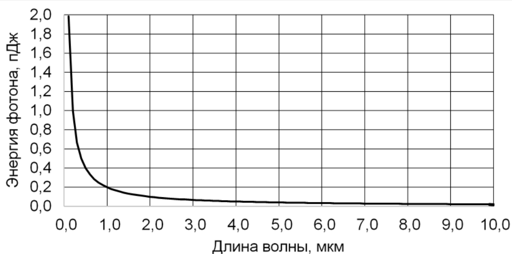
Рисунок 2.5 – Зависимость энергии фотона от длины волны излучения
