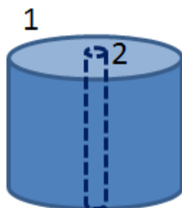
Рис. 22. Оболочка 1 размещена вокруг проводника 2 под напряжением, электрическое поле существует только между проводником и заземленной оболочкой
