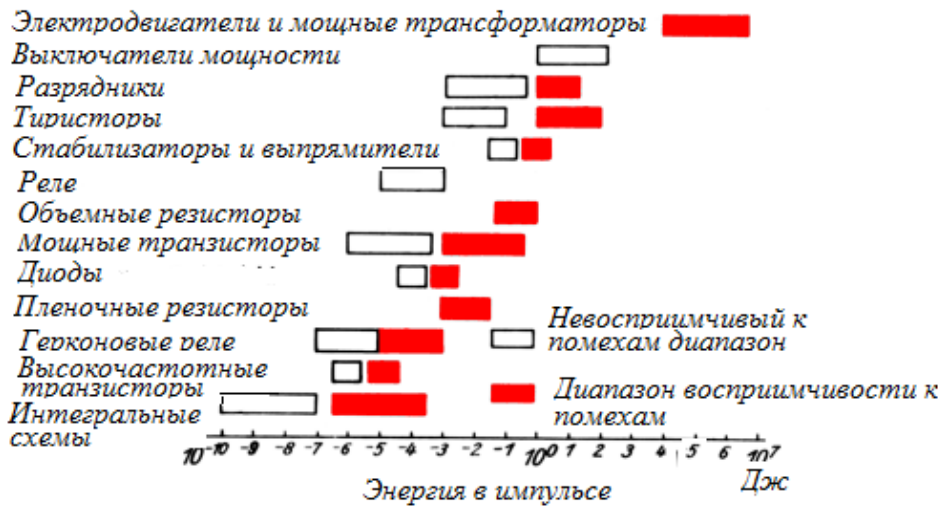
Рис. 10. Чувствительность к помехам различных устройств и электронных компонентов
