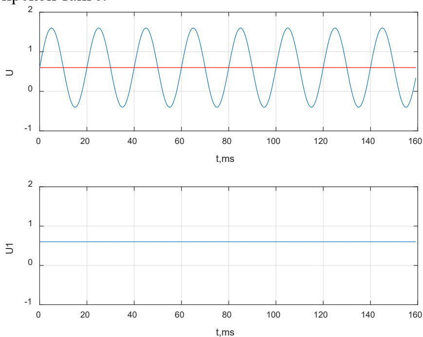
Рис. 15. Пример действия сетевой помехи на сигнал от датчика. На верхнем рисунке красная линия – сигнал от датчика, синяя – сетевая помеха. На нижнем – сигнал после подавления помехи
