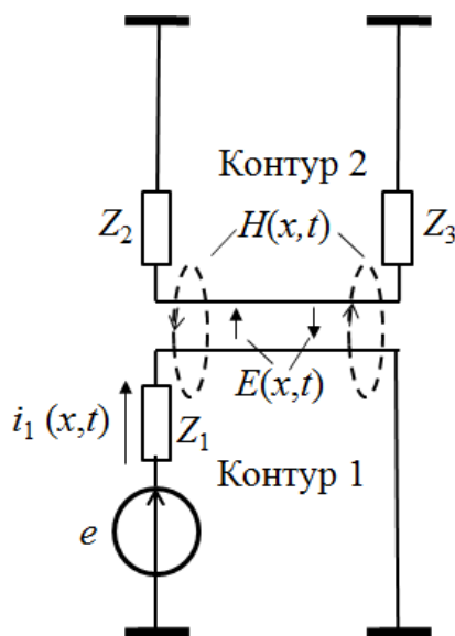
Рис. 42. Модель двух параллельных линий с общим обратным проводником («земля»)
