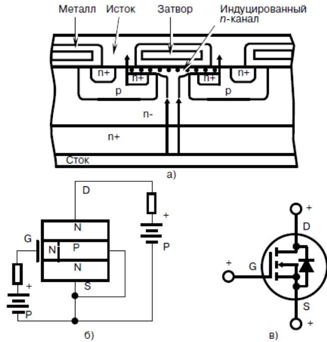
Рис. 8. МОП-транзистор с входящим в его структуру защитным («паразитным») диодом: а – структура, б – схема включения, в – схема включения паразитного диода [8]
