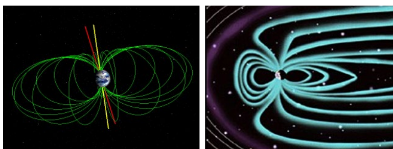
Рис. 3. Магнитное поле Земли: в спокойном состоянии (слева), после встречи с протуберанцем (справа)
