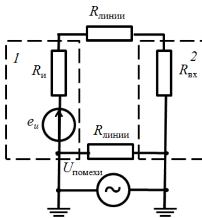
Рис. 38. Влияние контура заземления (многократное заземление) на помеху.
