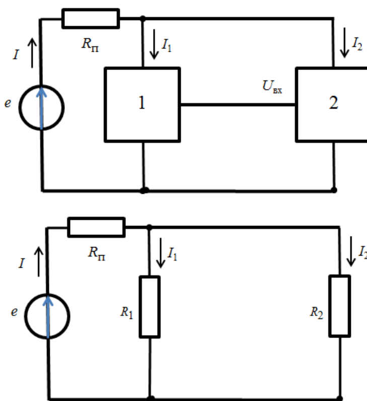
Рис. 37. Влияние общего проводника по цепи питания R_{\Pi} :
