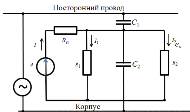
Рис. 39. Паразитная емкостная связь. C_1 и C_2 – паразитные емкости
