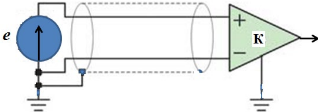
Рис. 57. Правильное заземление экрана. Соединяется с «землей» только в одной точке, у источника сигнала – датчика
