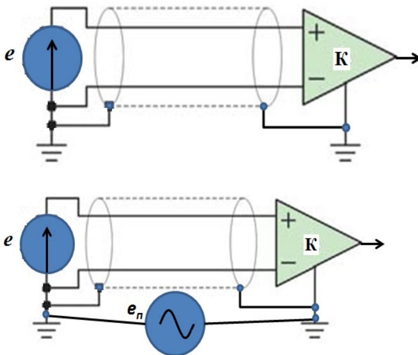
Рис. 56. Неправильное заземление экрана. Появляется паразитная ЭДС помехи e_n между двумя «землями», находящимися под разными потенциалами
