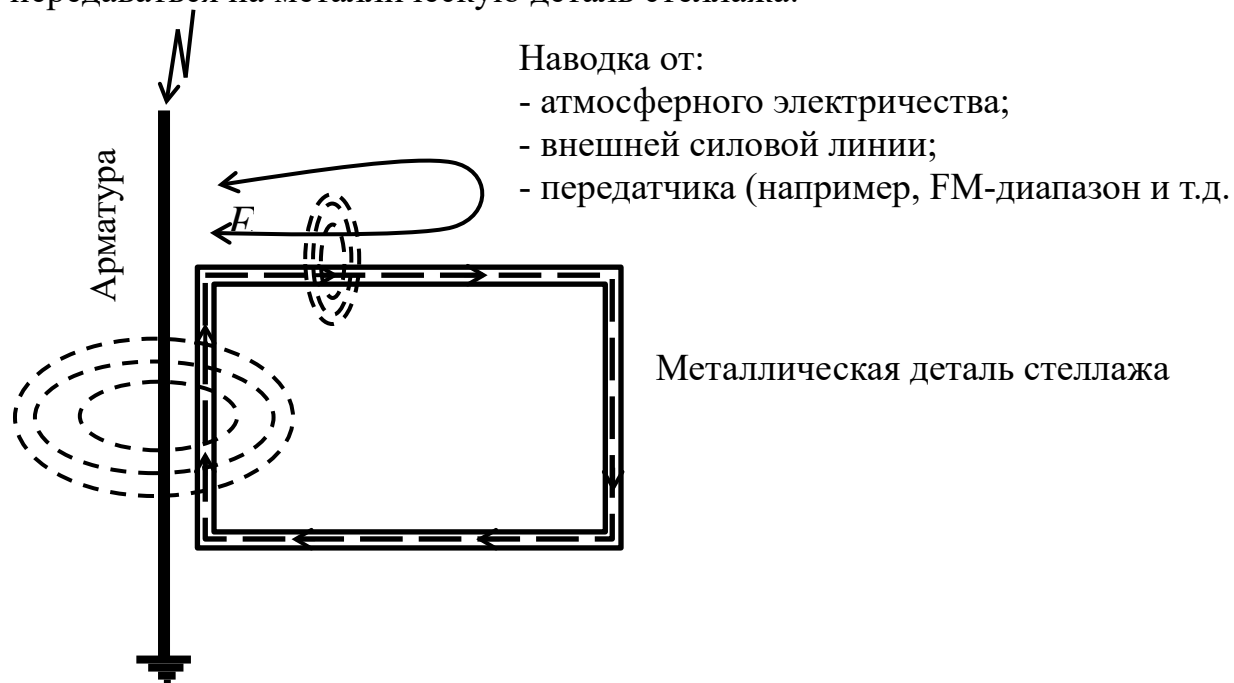
Рис. 28. Попадание помехи через арматуру здания я на металлическую деталь стеллажа
