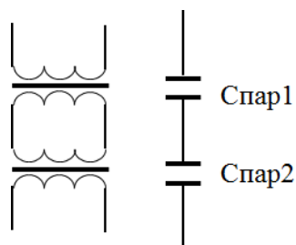
Рис. 55. Представление трансформаторов как паразитных емкостей C_{\text{спар}} . Если C_{\text{спар1}} = C_{\text{спар2}} = C_{\text{спар}} , то их последовательное соединение дает емкость C_{\text{спар}}/2 . Таким образом, уменьшается влияние паразитных емкостей
