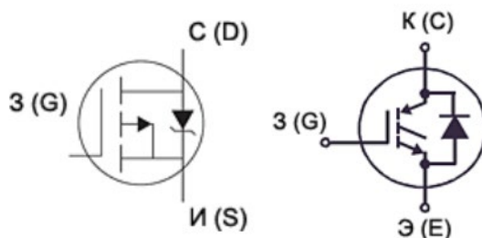
Рис. 52. Условные обозначения МОП (слева) и БТИЗ (справа) транзисторов
