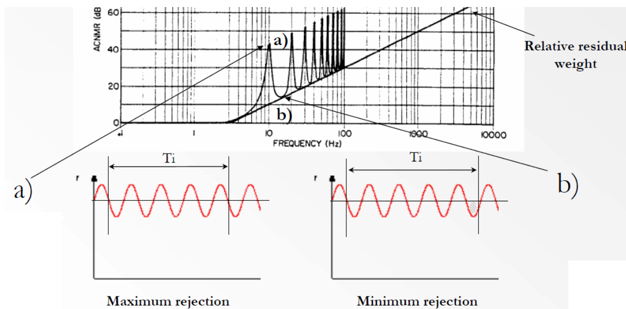
Рис. 14. Коэффициент подавления помехи нормального вида в зависимости от частоты [9]. Иллюстрируется максимальное подавление, когда не период измерения приходится целое число периодов помехи (четное число полупериодов), рисунок 12а, и минимальное, когда число периодов помехи нецелое (нечетное число полупериодов), рисунок 12б
