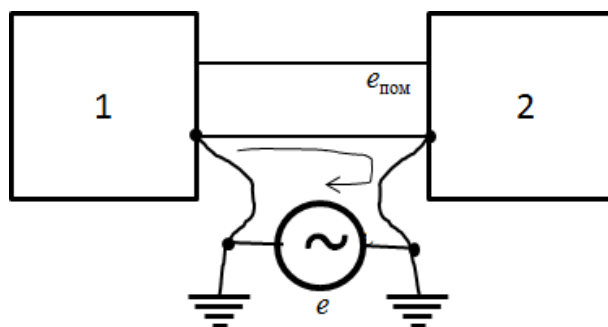
Рис. 29. Заземление в двух разных точках. Стрелкой показан ток в контуре заземления
