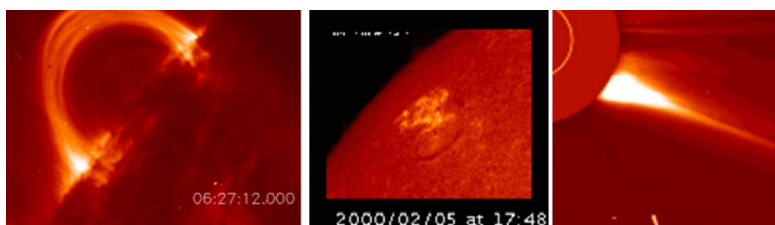
Рис. 2. Солнечные протуберанцы
