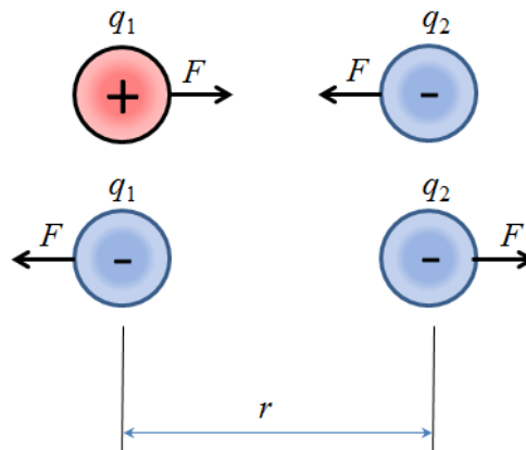
Рис. 18. Два электрически заряженных тела с зарядами q_1, q_2 [Кл] на расстоянии r [м] в пространстве притягиваются или отталкиваются друг от друга с силой F [Н] в зависимости от соотношения полярностей
