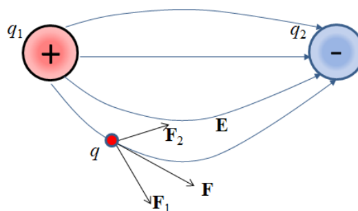
Рис. 19. Для каждой точки пространства описывается действие силы F , вызванной взаимодействием сил, исходящих от большого числа других зарядов
