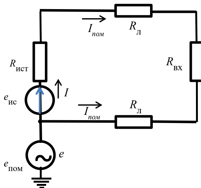
Рис. 44. Синфазная помеха. Помеха в двух сигнальных проводниках действует в одном направлении
