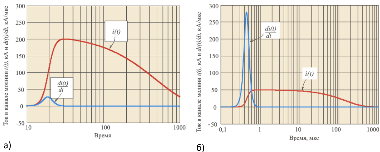
Рис. 6. Зависимость тока первого (а) и второго (б) импульса молнии и его производной от времени [3, 4]
