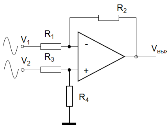
Рис. 51. Дифференциальный усилитель
